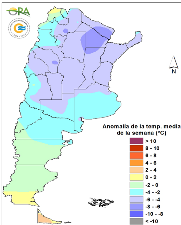
Anomalía de la temperatura media de la semana del 21/08/2024 al 27/08/2024
