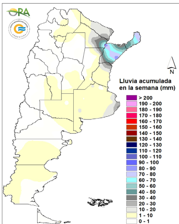
Precipitaciones acumuladas en la semana del 21/08/2024 al 27/08/2024
